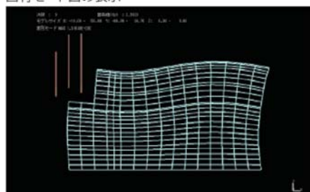
モード図
