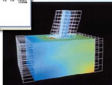
変形+応力
