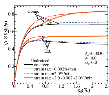
(a) 圧縮および伸張試験のひずみ速度効果
