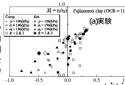
図-5 正規圧密粘土の応力比~ひずみ増分比関係
