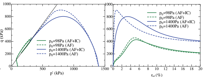
(b) 非排水試験の有効応力経路と応力~ひずみ関係 図-4 構造化した粘土の解析結果
