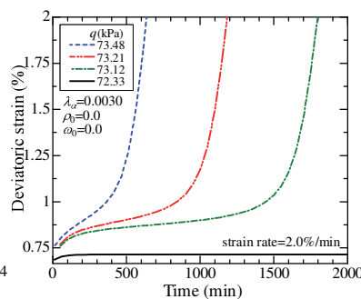
(b) 非排水クリープ曲線
