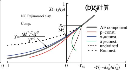
図-5 正規圧密粘土の応力比~ひずみ増分比関係
