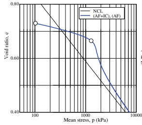
(a) 等方圧縮試験の圧密曲線
