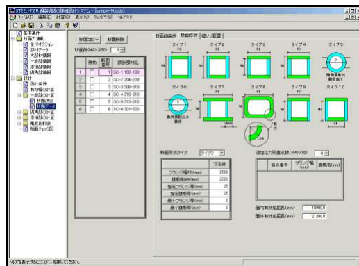
断面設計
