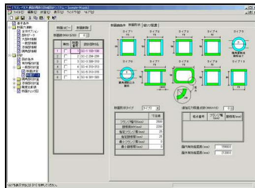
断面設計
