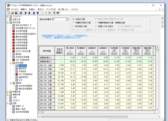
設計計算／設計結果－主桁設計
