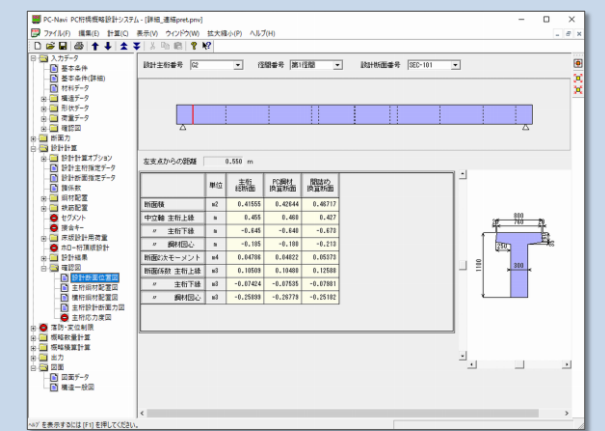
設計計算／確認図－設計断面位置図
