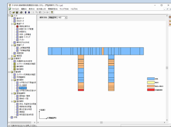
計算結果／静的解析－塑性域図
