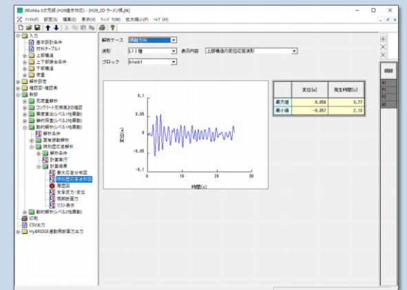
新設／動的解析(レベル 1)－時刻歴応答波形図
