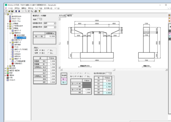
入力－下部構造－橋脚形状－ラーメン式橋脚
