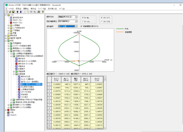
地震時保有水平耐力法－計算結果 －軸力-曲げモーメント相関関係
