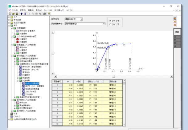
新設／静的照査(レベル 2)－Kh- \delta 、P- \delta 関係図
