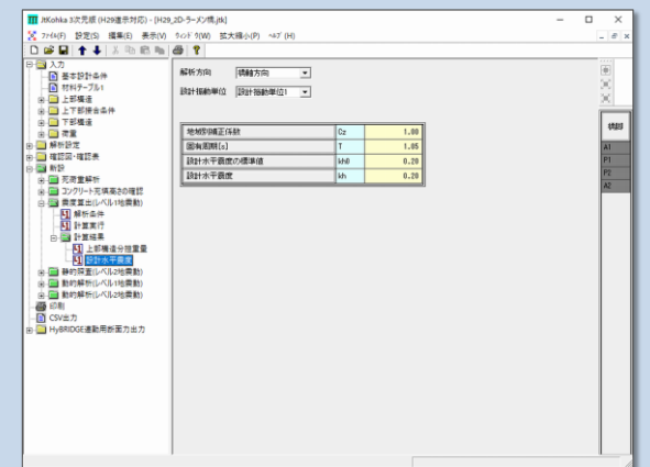
新設／震度算出(レベル 1)－設計水平震度
