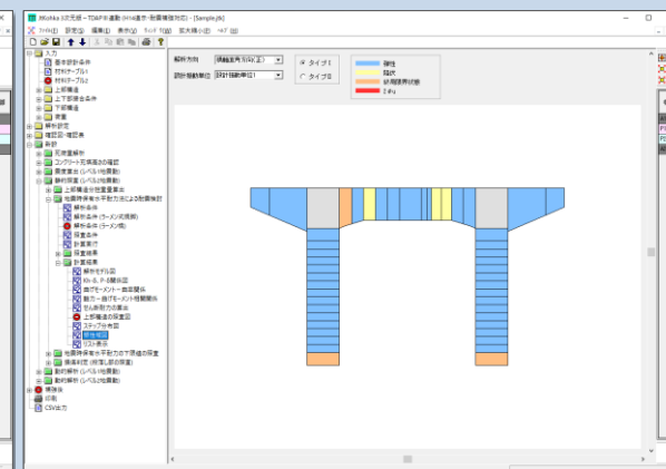
地震時保有水平耐力法－計算結果 －塑性域図
