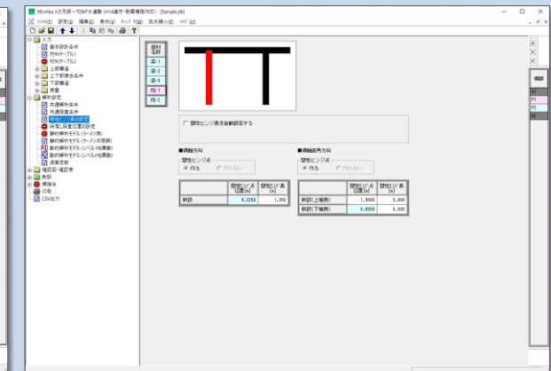
解析設定 - 塑性ヒンジ長の設定
