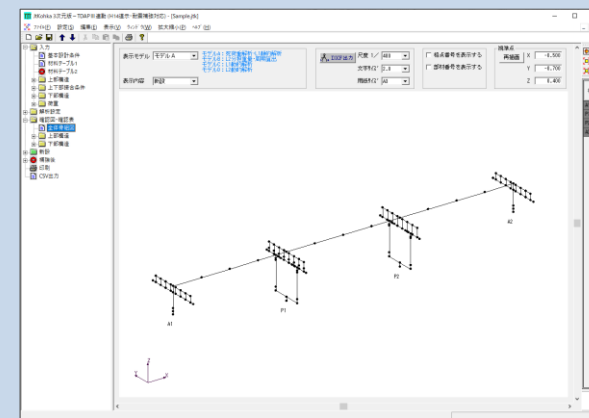
確認図・確認表 / 全体骨組図
