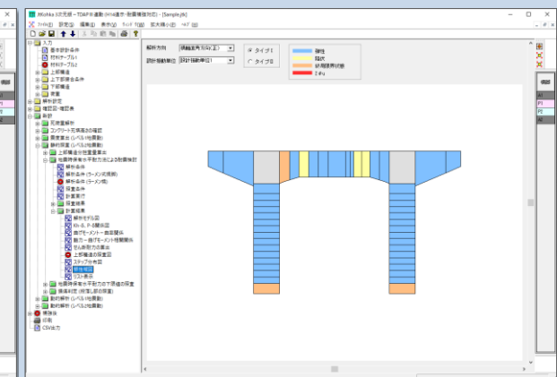
地震時保有水平耐力法 - 計算結果 - 塑性域図
