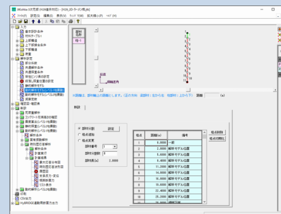
解析設定／動的解析モデル(レベル 1 地震動)
