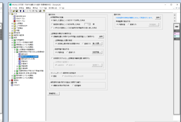
地震時保有水平耐力法 - 解析条件 (RC-ラーメン橋脚)
