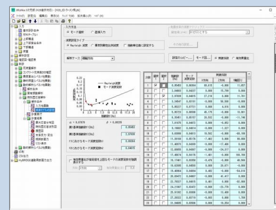
新設／動的解析(レベル 1) - 時刻歴応答解析
