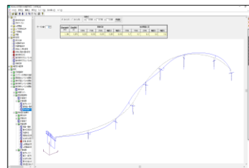
動的解析／固有振動モード図
