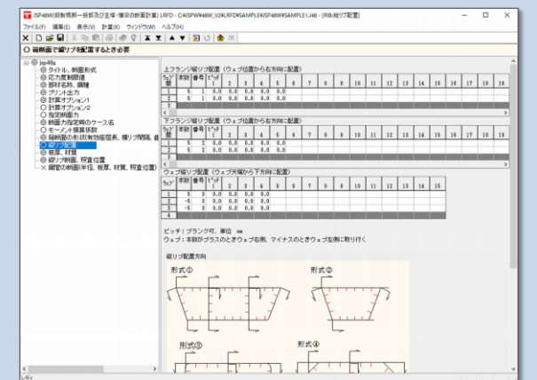
縦リブ配置
