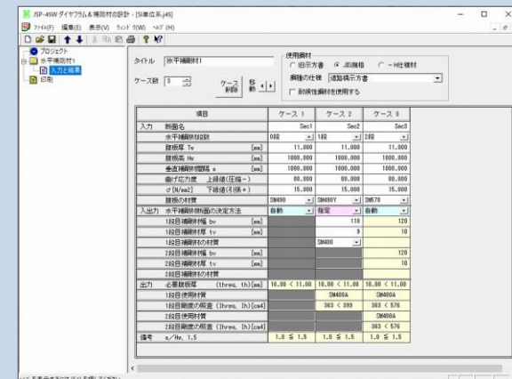
水平補剛材 1 / 入力と結果
