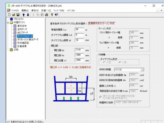
中間ダイア 1 / ダイヤフラムデータ
