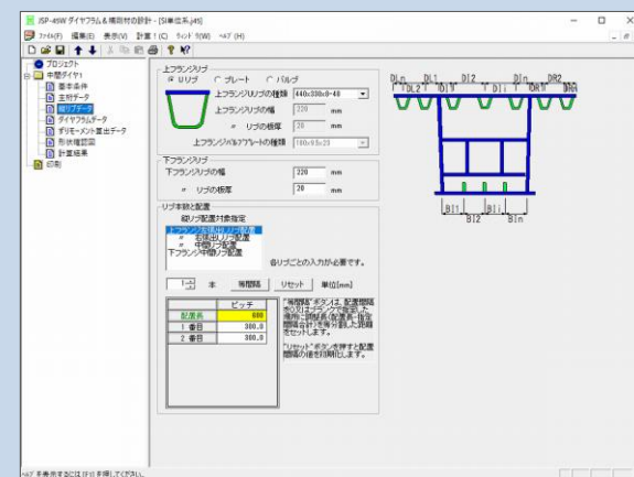
中間ダイア 1 / 縦リブデータ
