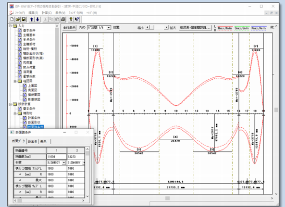
設計計算／補剛桁－断面諸条件
