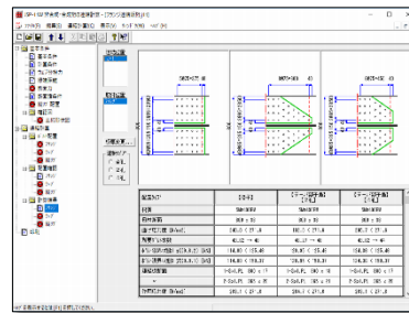
連結計算／計算結果－フランジ
