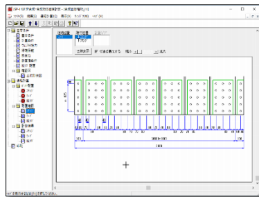
連結計算／配置確認－フランジ
