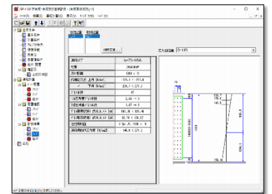
連結計算／計算結果－ウェブ
