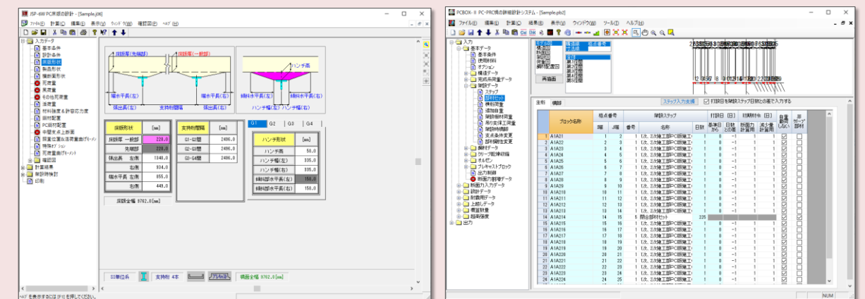
入力データ(JSP-6W)／床版形状
