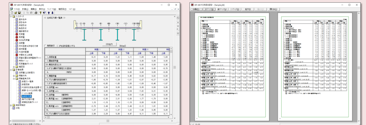
計算結果／橋軸直角方向－合成応力度
