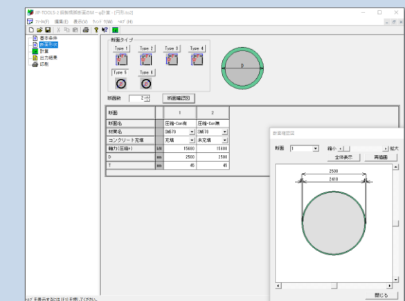
断面形状(円形)
