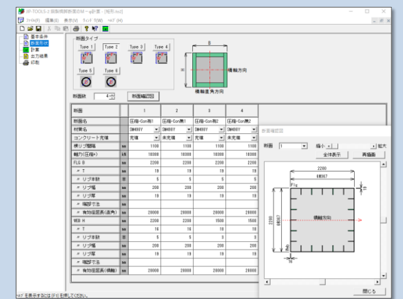
断面形状(矩形)
