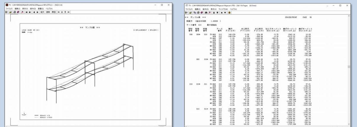
計算結果／変形図
