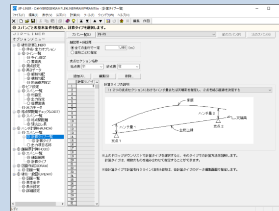
ハンチ計算/スパン一覧-計算タイプ一覧
