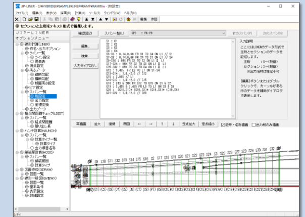
線形計算/スパン一覧-桁設定
